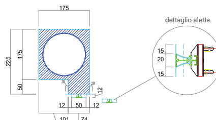
Dettaglio PS2F altezza 50 mm con attacco L
