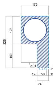
Dettaglio PSDM altezza 50 mm con attacco L
