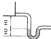
Allacciamento scarico condensa
